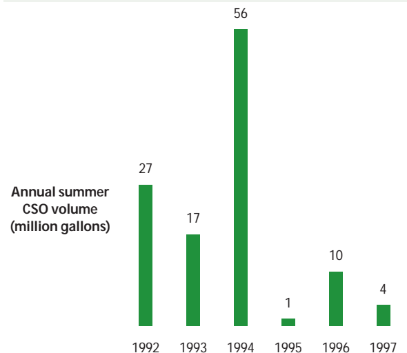
Summer CSO Volume Reductions, 1992—1997
